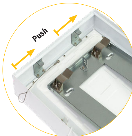
Einfach montieren mit Montageplatten und Push-Federarretierung für alle Leuchtengrößen
